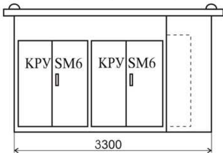
Поглед страна средно напрежение
